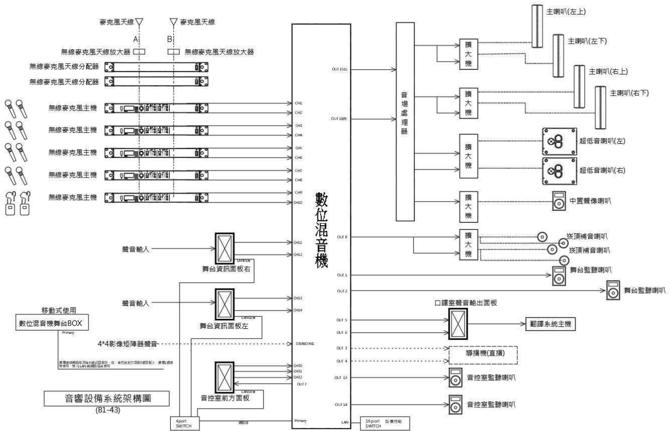
音響設備系統圖
